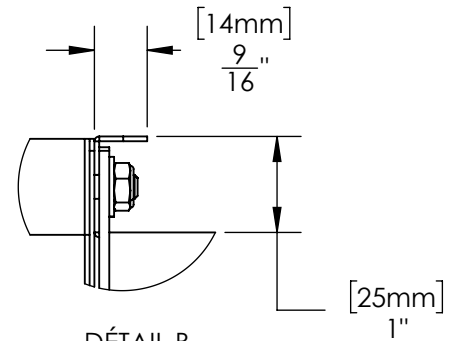
DÉTAIL B ECHELLE 1 : 2
